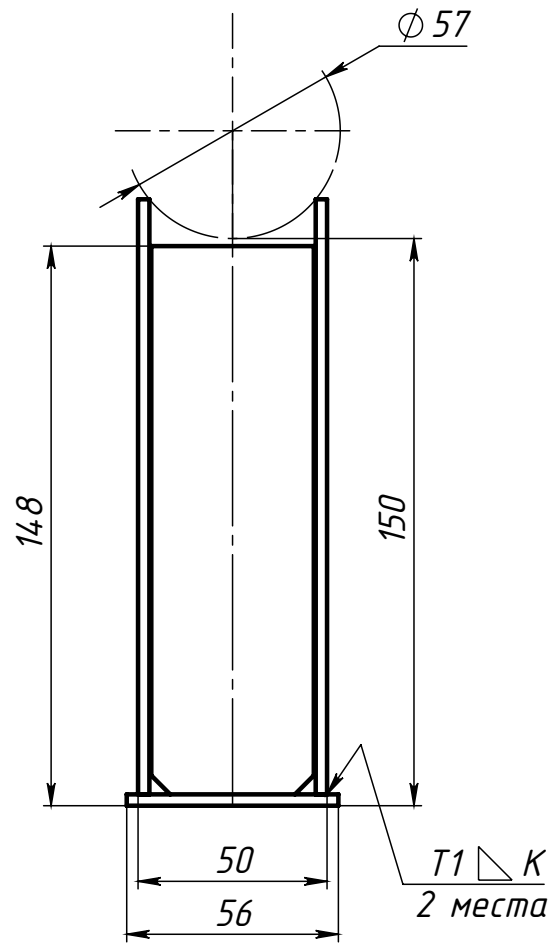
Поз.2 (Редро)
