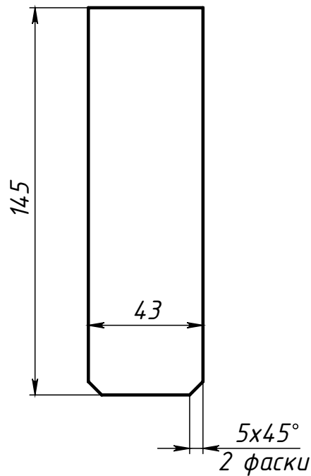
Поз.2 (Редро)
